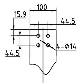
L.V. TERMINAL
